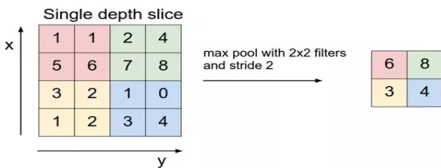
Fig 5: Max Pooling Layer
