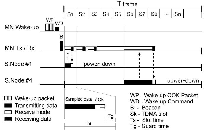
Fig. 4. TDMA frame
