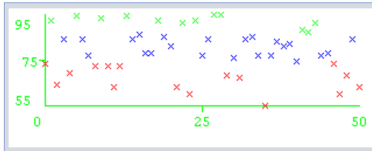
Fig. 2. Clustering
