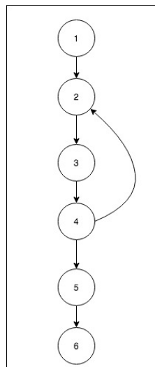
Fig. 5. Login Flowgraph
