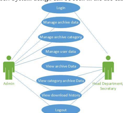
Fig. 3. Usecase Diagram
