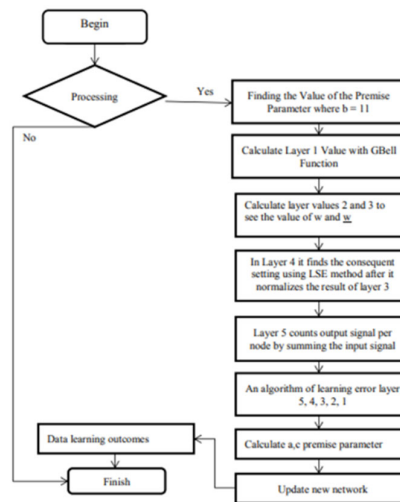
Fig 3. ANFIS Flowchart
