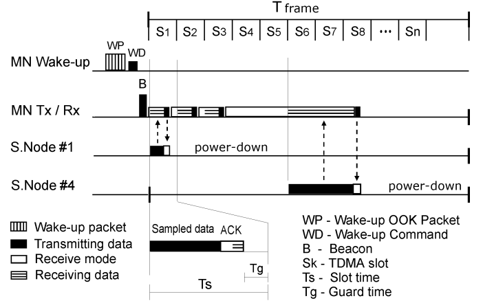
Fig. 4. TDMA frame
