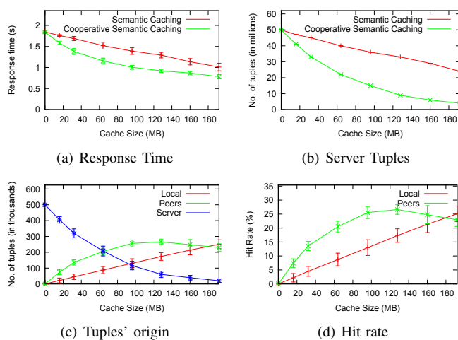
Fig. 12. Cache Size 1D
