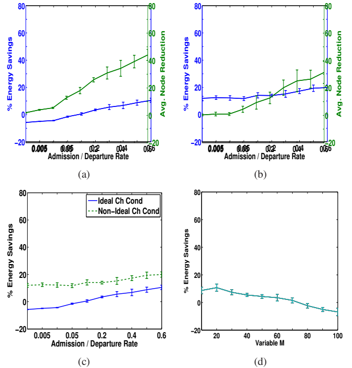
Fig. 2. Optimal Scheme
